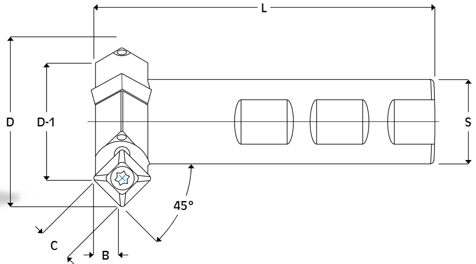
Tool Info.
