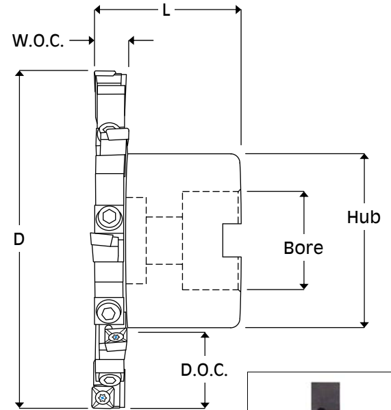
R.H. Cartridge
