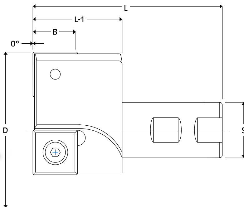
Tool Info.
