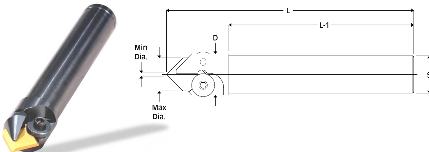
Tool Info.
