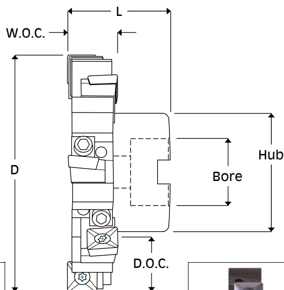
R.H. Cartridge
