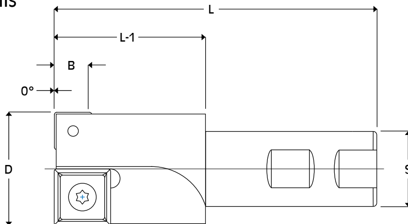
Tool Info.
