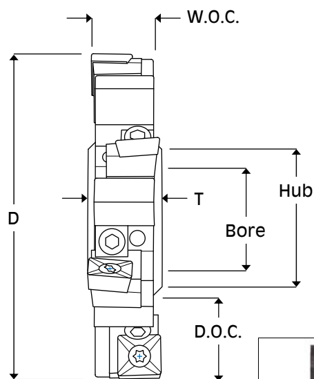
R.H. Cartridge
